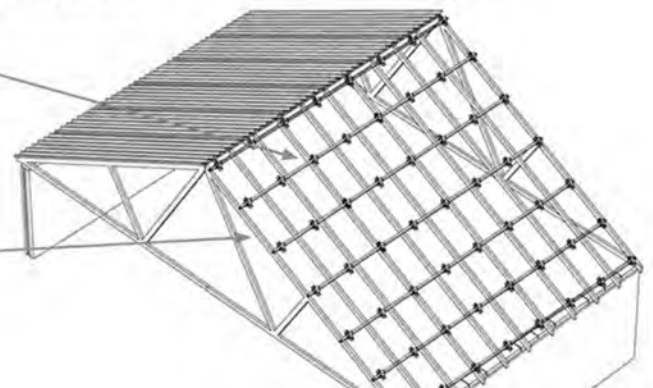
Buttée inférieure
